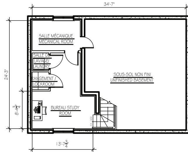
PLAN DU SOUS-SOL - BASEMENT FLOOR PLAN
