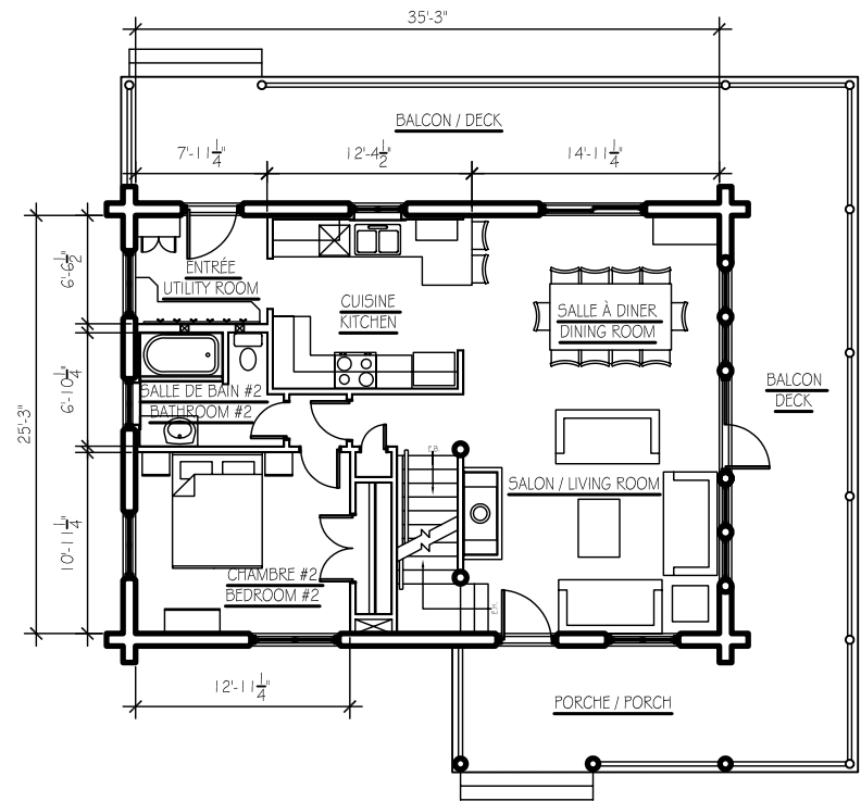
PLAN DU REZ-DE-CHAUSSÉE - MAIN FLOOR PLAN
