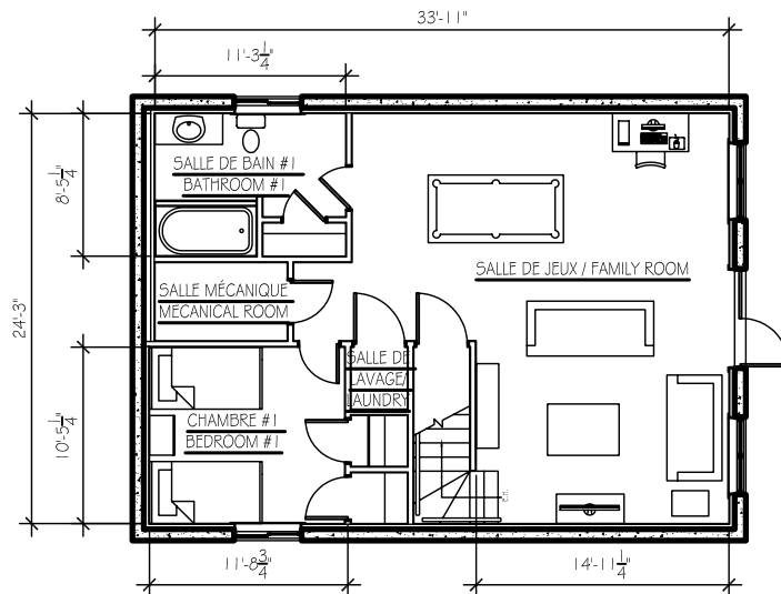
PLAN DU SOUS-SOL - BASEMENT FLOOR PLAN
