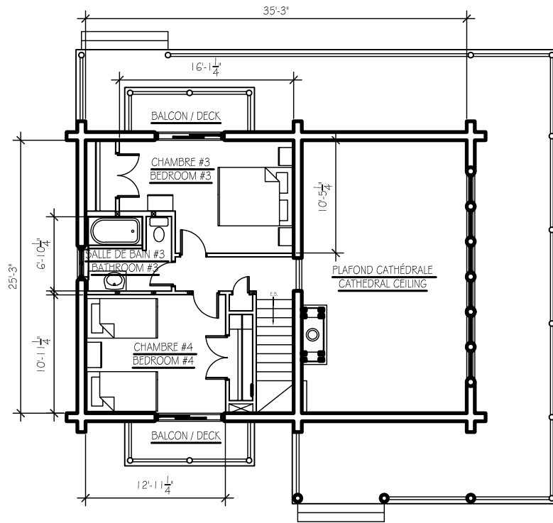
PLAN DE L'ÉTAGE - UPPER FLOOR PLAN
