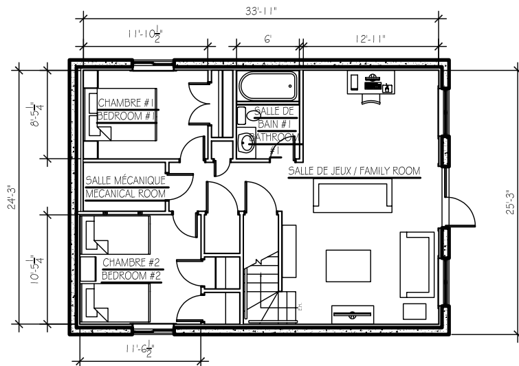
PLAN DU SOUS-SOL - BASEMENT FLOOR PLAN
